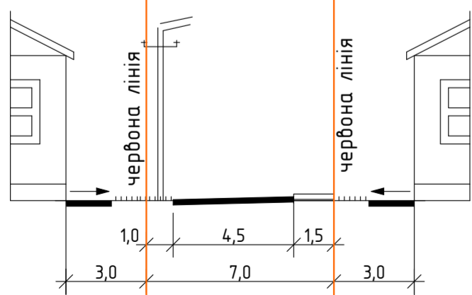
Креслення поперечних профілів вулиць М 1:200 проєктна вулиця
